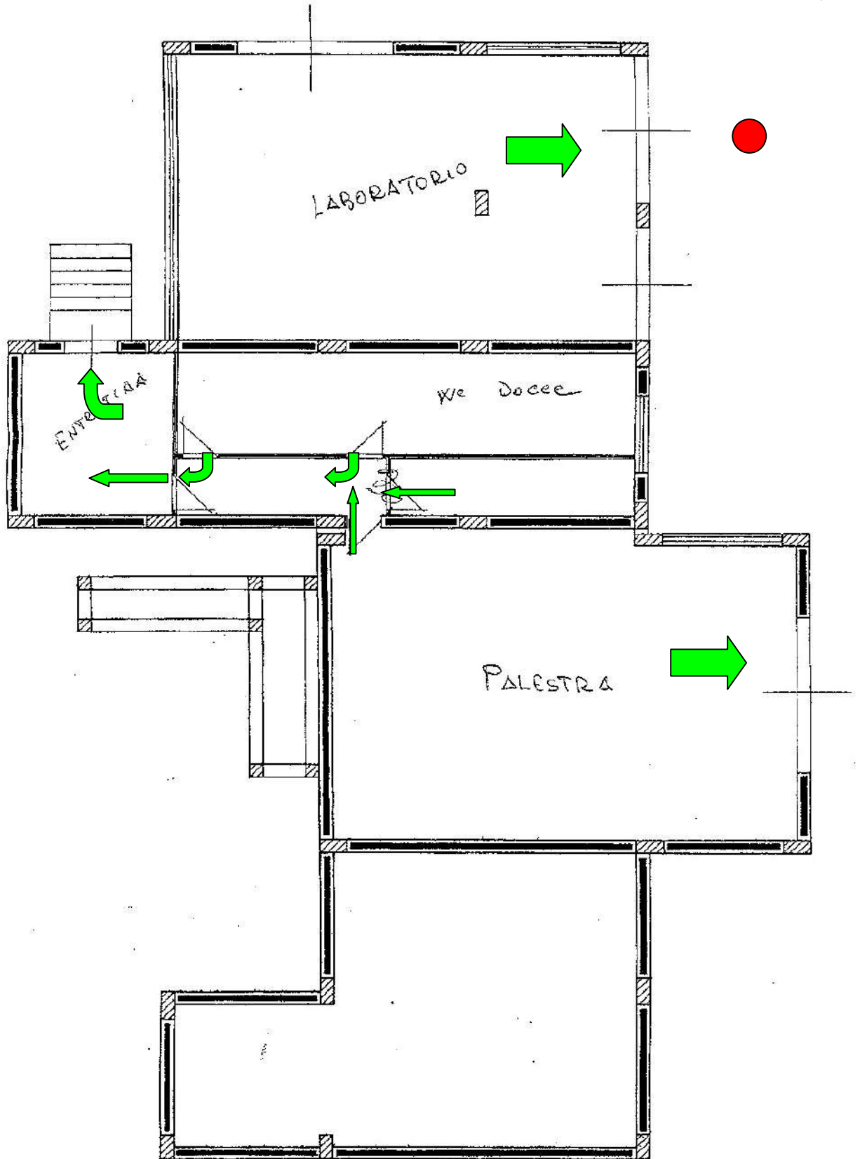
Scuola Media Francavilla – Piano Seminterrato
